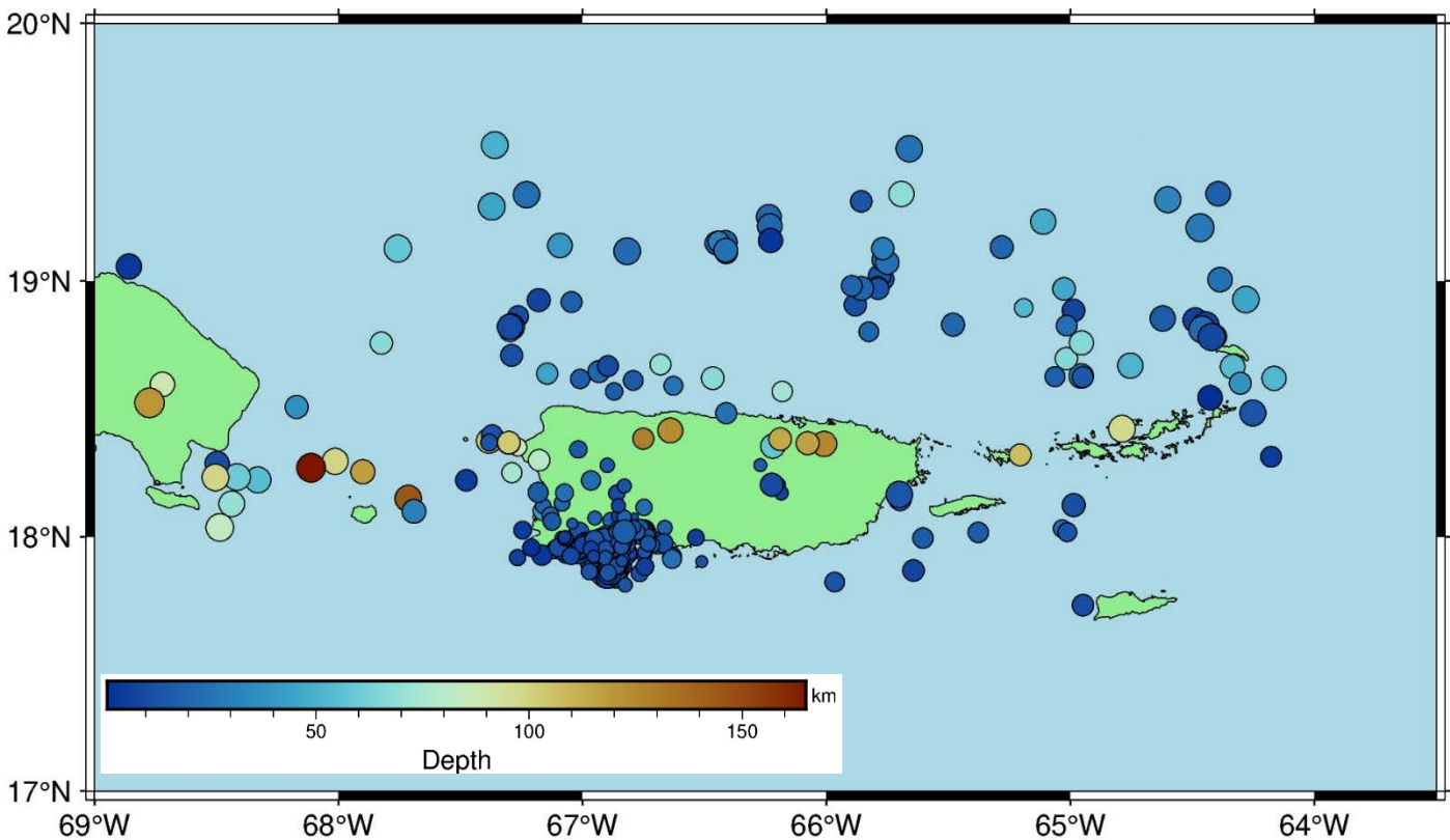
Figura 1. Mapa epicentral de los sismos localizados en la Región de Puerto Rico e Islas Vírgenes por la RSPR para el mes de agosto de 2022 (RSPR-UPRM).
